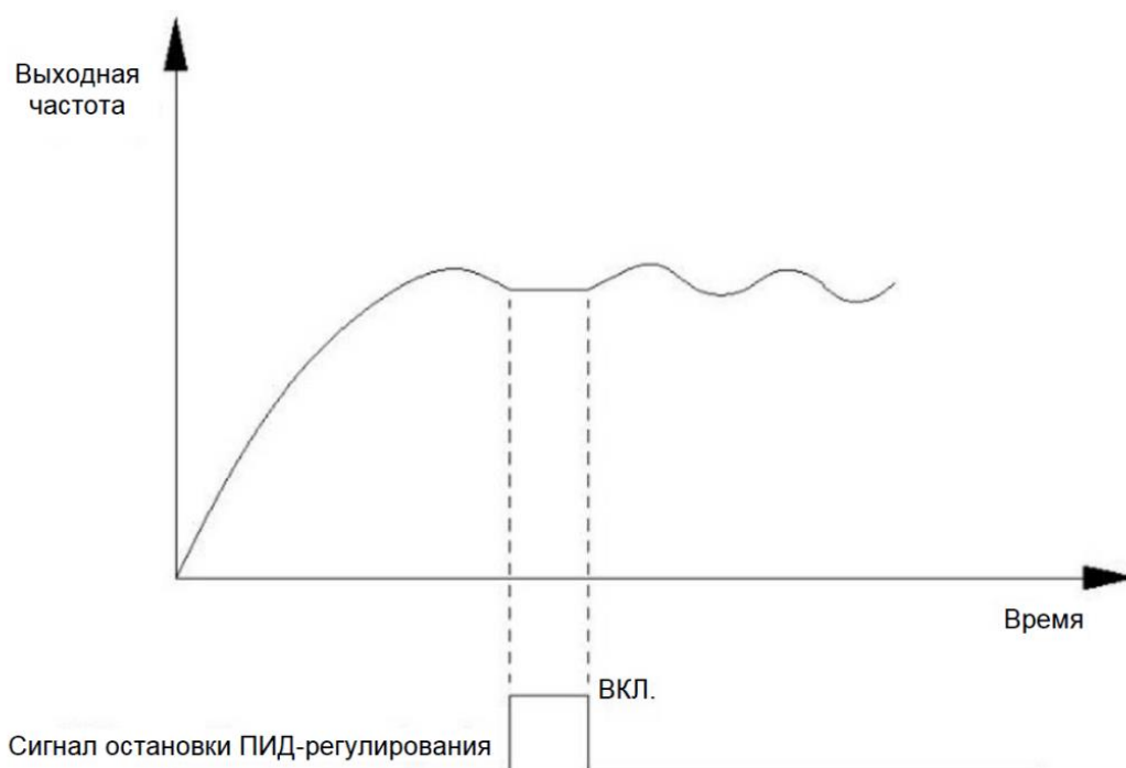
Рисунок 5-10 Схематическая диаграмма приостановки ПИД-регулирования
