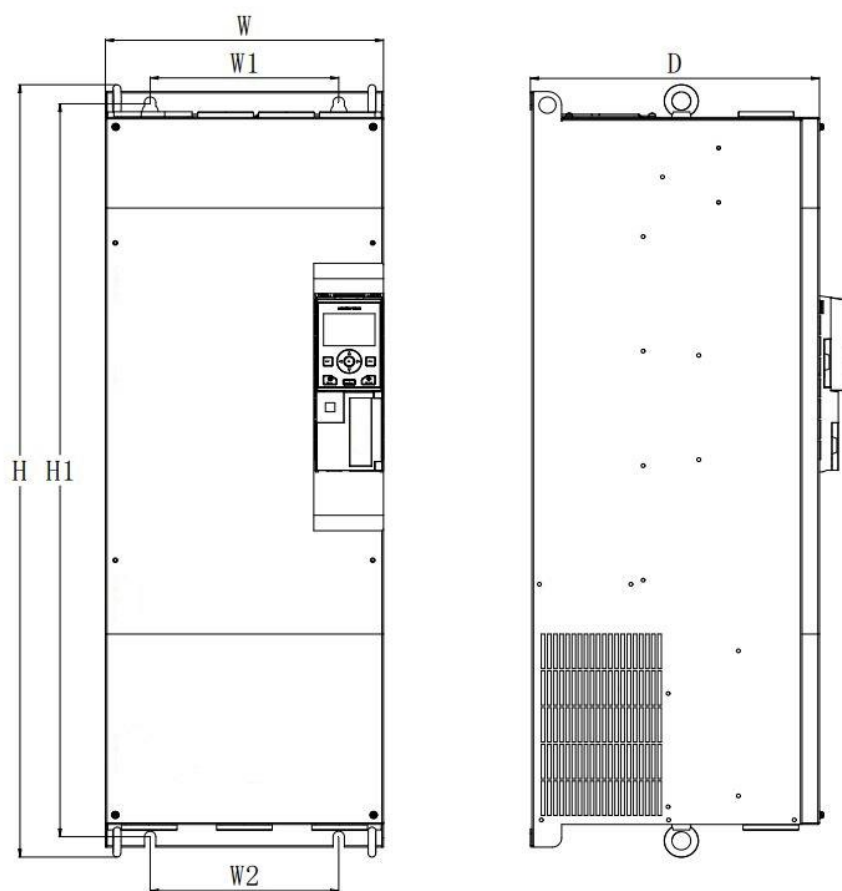
Рис. 1-5 Установочные размеры IMD373U43E1 ~ IMD204U43E1 (37кВт ~ 200кВт)
