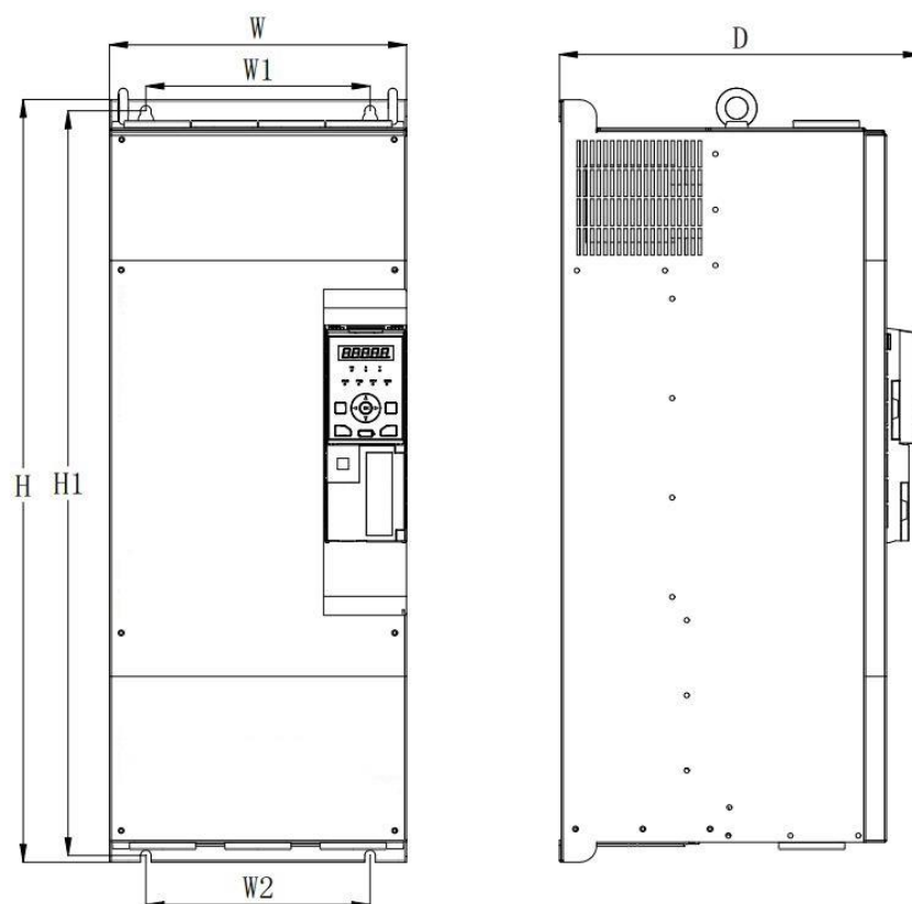
Рис. 1-4 Установочные размеры IMD183U43E1 ~ IMD303U43E1 (18.5кВт ~ 30кВт)
