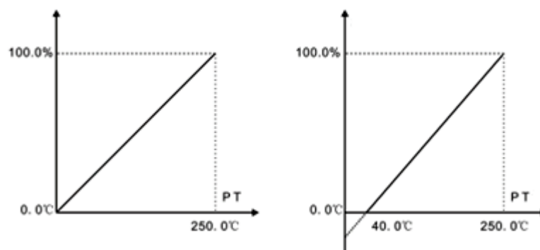
Рис. 5-19 Пример настройки температурной кривой
