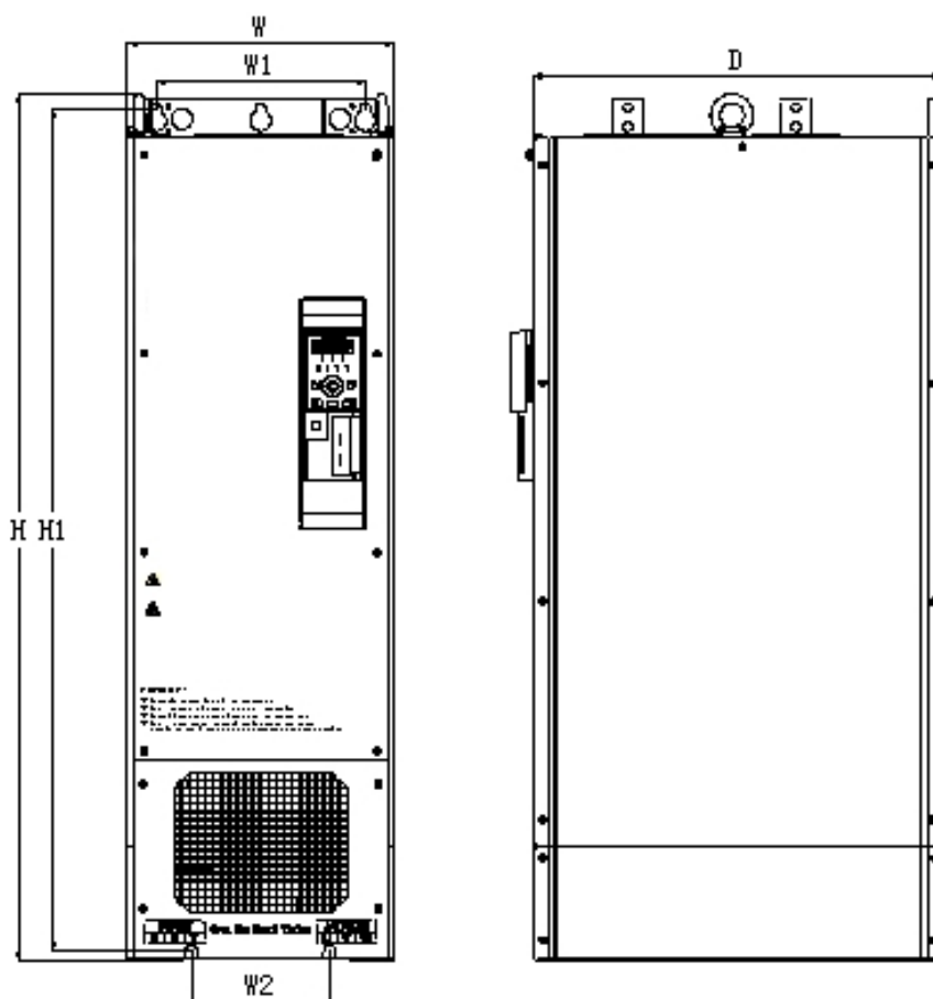
Рис. 1-6 Установочные размеры IMD224U43E1 ~ IMD404U43E (220кВт ~ 450кВт)
