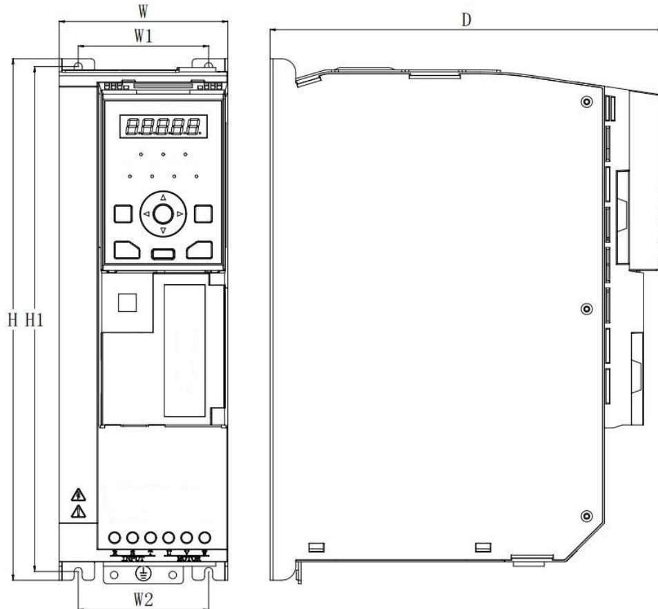
Рис. 1-3 Установочные размеры IMD552U43E1 (5,5кВт) и ниже
