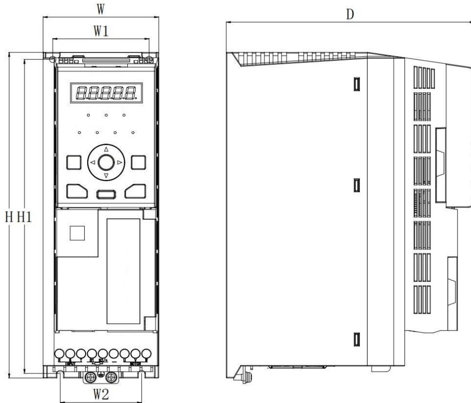
Рис. 1-3 Установочные размеры IMD552U43E1 (5,5кВт) и ниже
